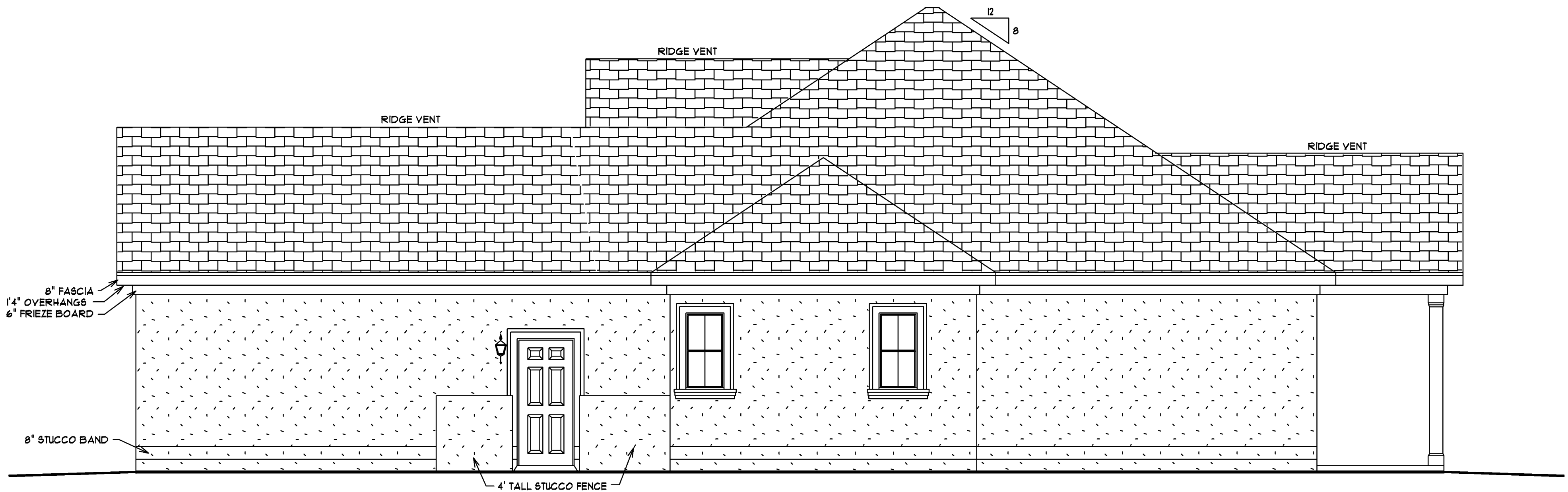
RIGHT ELEVATION
