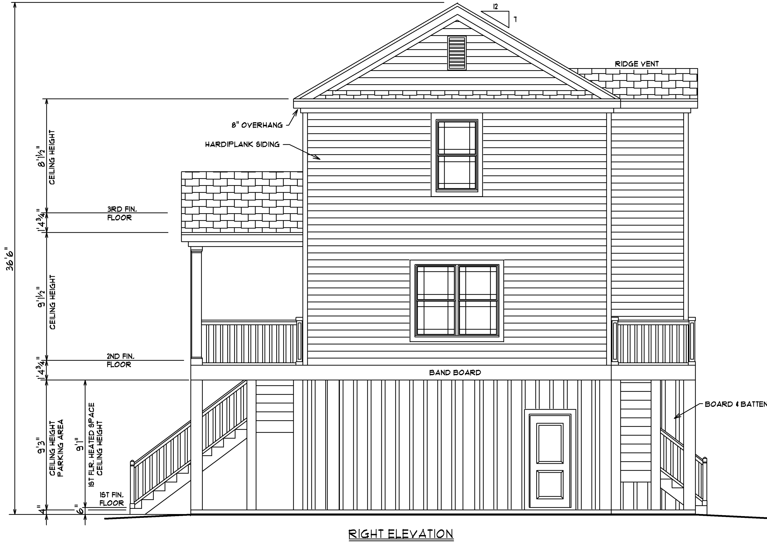
RIGHT ELEVATION
